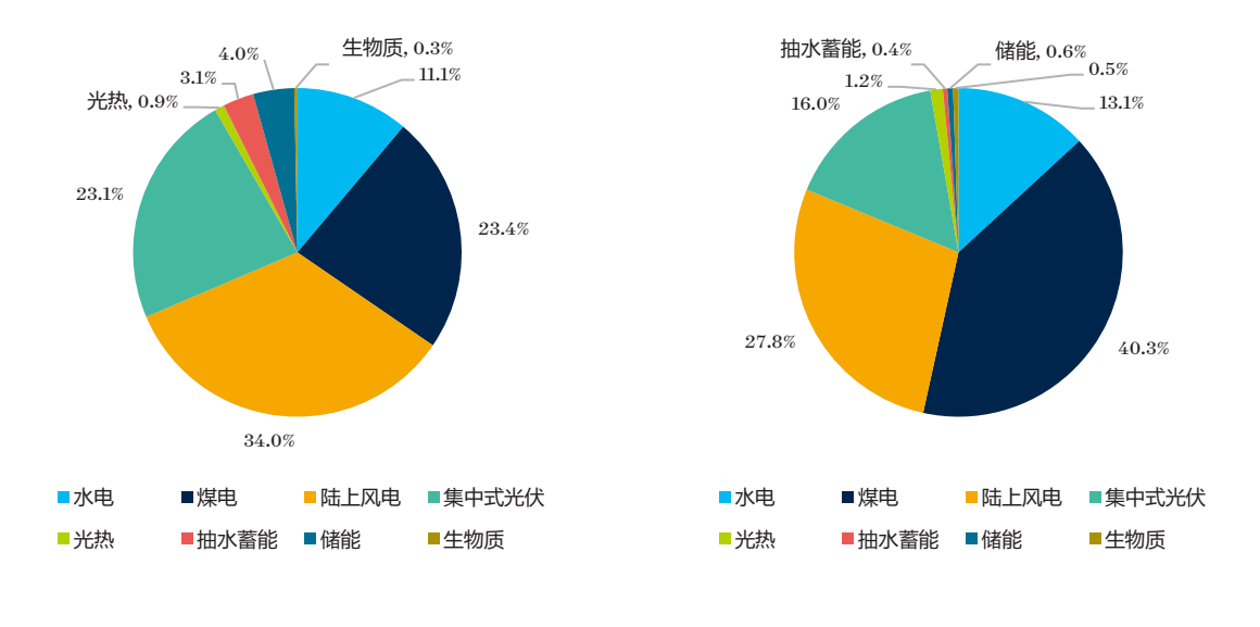
图3-9 甘肃省2030年各类电源装机占比（左）及发电量占比（右）
