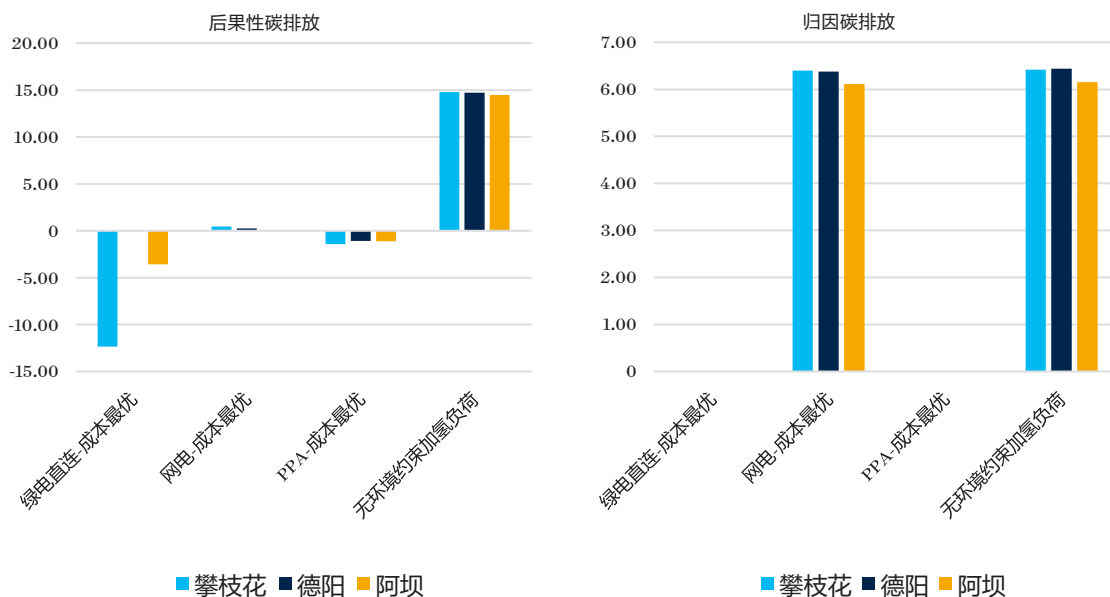
图3-7 攀枝花市、德阳市、阿坝州各制氢场景后果性碳排放（左）及归因碳排放对比（右）（ \text{tCO}_2/\text{tH}_2 ）
